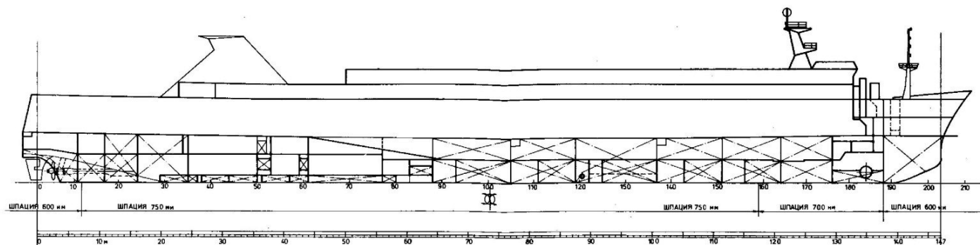
НИЖНЯЯ ПАЛУБА
